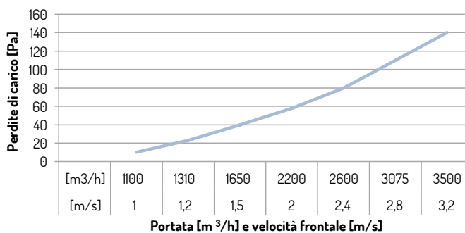
Modulo CARBOX55_6
