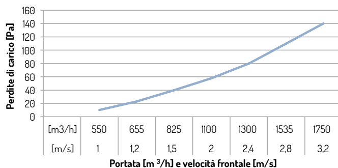
Modulo CARBOX27_6
